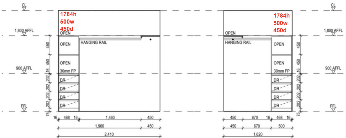
01 WIR INTERNAL ELEVATION SCALE: 1:50
