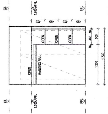
G1 BED 3 ROBE INTERNAL ELEVATION SCALE: 1:50
