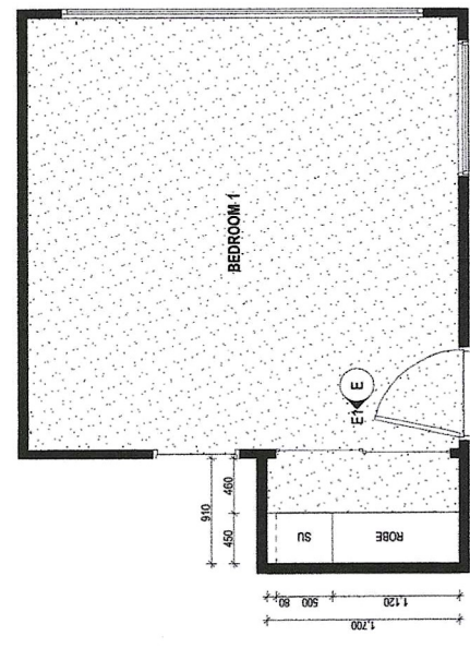
E BED 1 ROBE DETAIL PLAN SCALE: 1:50
