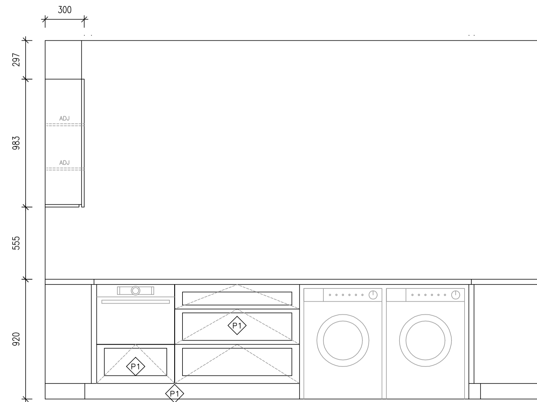
ELEVATION B
