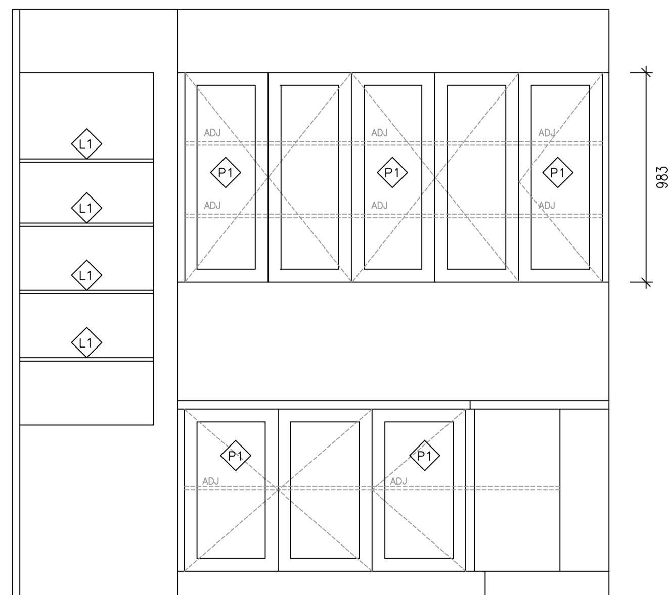
ELEVATION A
