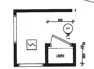
L LINEN DETAIL PLAN SCALE: 1:50
