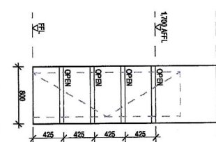
11 LINEN INTERNAL ELEVATION SCALE: 1:50
