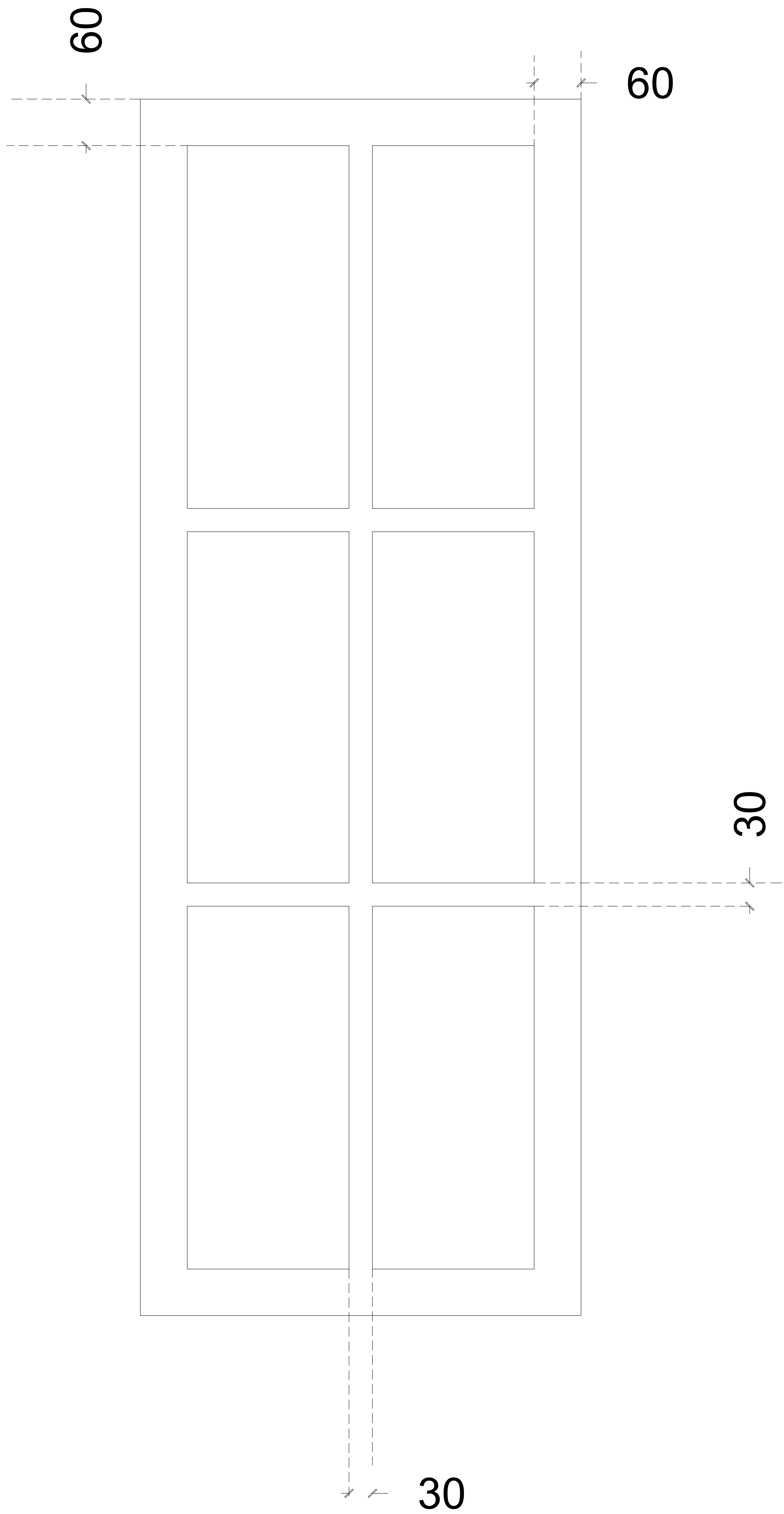
Cab # 2,3 door detail
