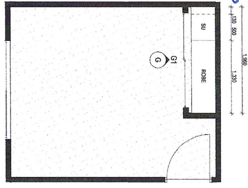
G BED 2 ROBE DETAIL PLAN SCALE: 1:50
