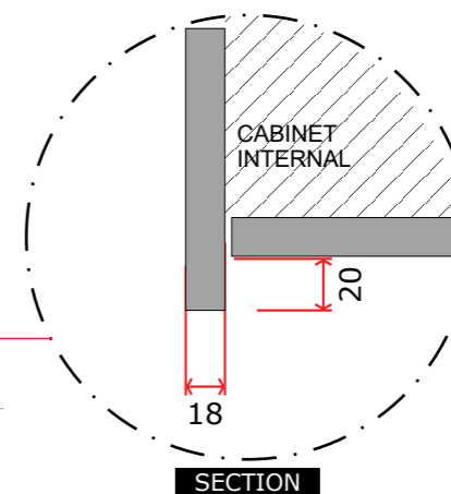
DET. 01 DOOR HANGDOWN FINGERPULL HANDLE SCALE: 1:5
