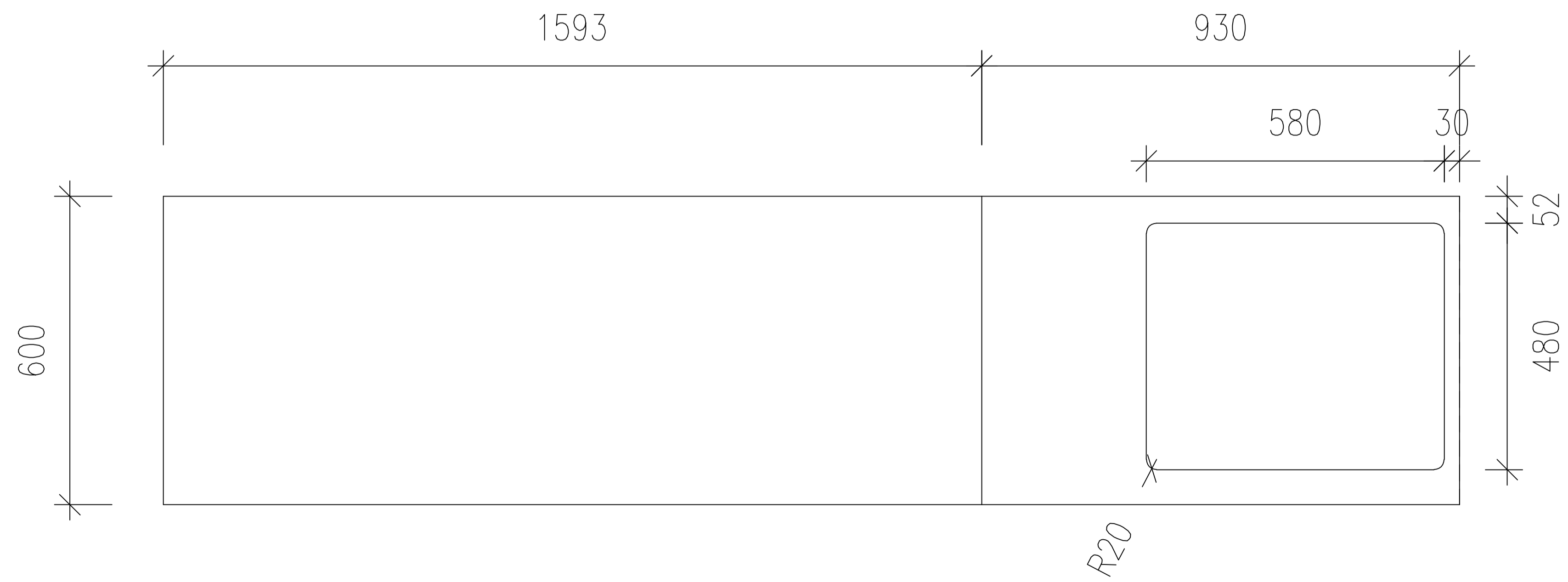
3mm MDF Template
